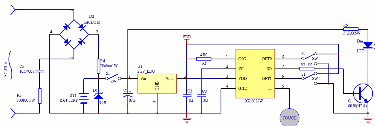
图 2、使用充电电池供电时的应用电路
